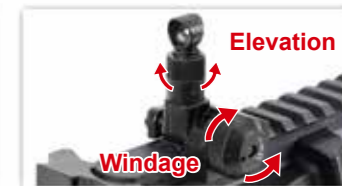
偏差つまみ (左/右 調整) 仰角つまみ (上/下 調整)
